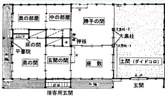
建築当初の平面図
