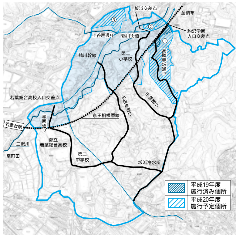
図 稲城市公共下水道事業(汚水) 第3期事業予定区域
