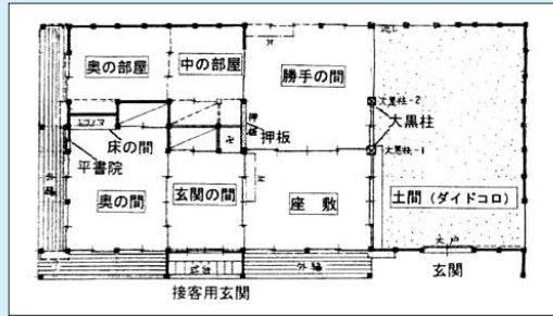
▲建築当初の平面図
